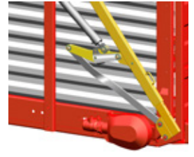
Einstellbare Rückwandstrebe
