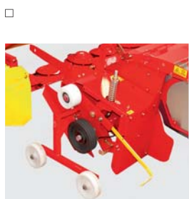
Fahrwerk für Aufbereiter
