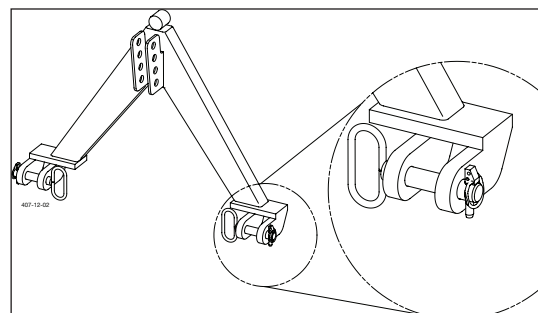
Klappvorstecker innen (Abb 1)
