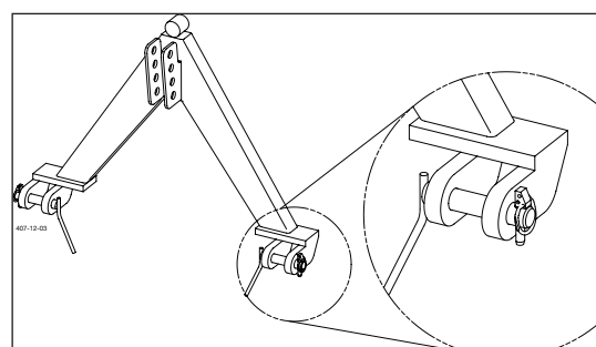
Klappvorstecker außen (Abb 3)
