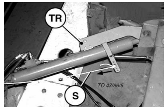
Transportstellung
