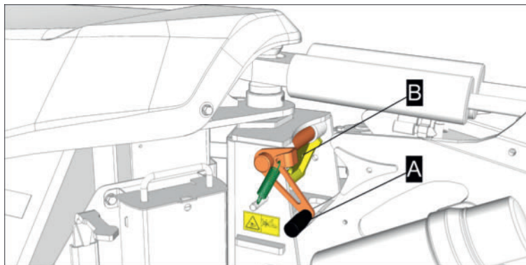
Sicherheitsklappe an der linken Mäheinheit in entsperrter Position
