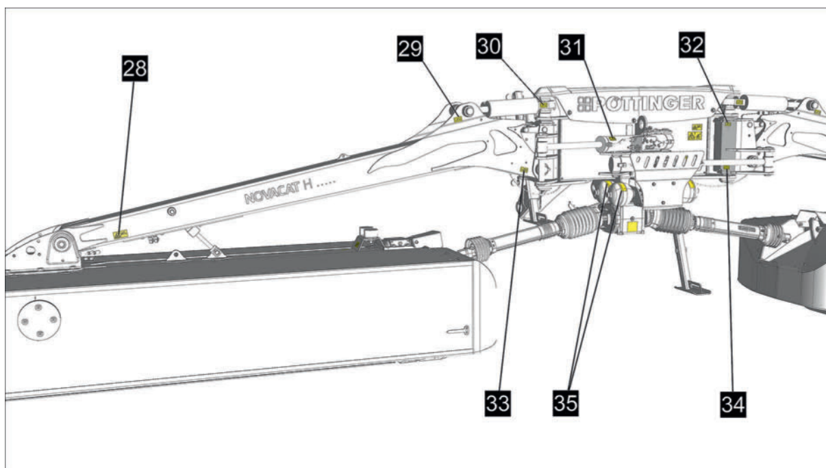
Linker Ausleger und Anbaurahmen hinten.
