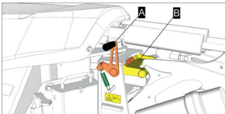
Sicherheitsklappe an der linken Mäheinheit in gesperrte Position eingeschwenkt
