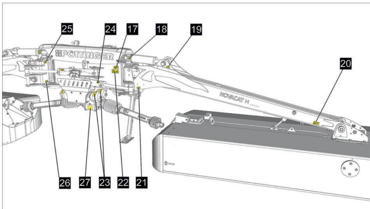
Rechter Ausleger und Anbaurahmen hinten.
