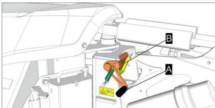
Linker Ausleger: Sicherungsklappe (B) in entspernter Position
