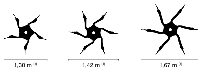
(1) Diámetro rotor
