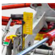
Ajuste de altura del rotor hidráulico
