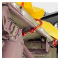
Hydraulische Seitenschutzklappung
