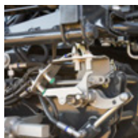
Hydraulische schakeling voor messenvoorkeuze
