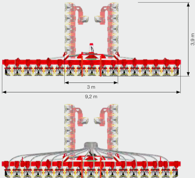
Levitysjärjestelmä 16 ulostulolla ja erillisillä letkuilla
