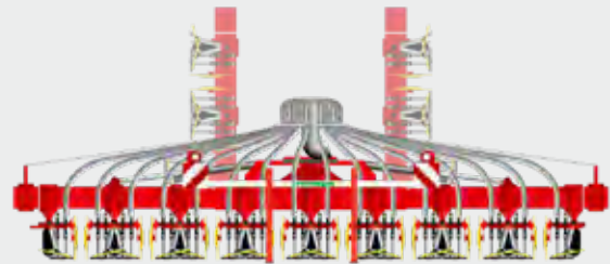
Levitysjärjestelmä 16 ulostulolla ja kaksoisletkuilla
