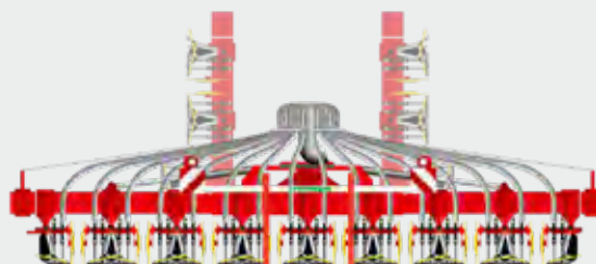
Sistema di distribuzione con 16 scarichi e tubazioni doppie
