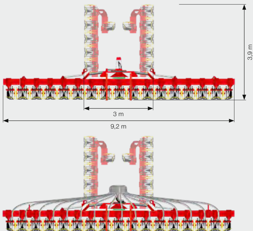
Sistema di distribuzione con 16 scarichi e tubazioni singole
