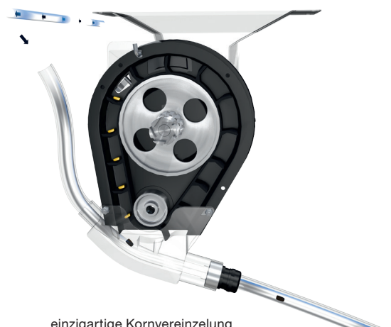
einzigartige Kornvereinzlung
